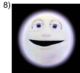
moon
