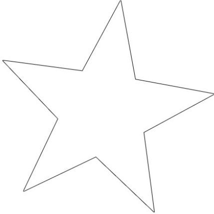
star
