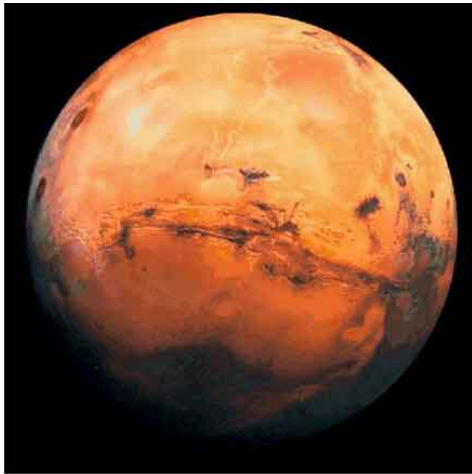
Mars
